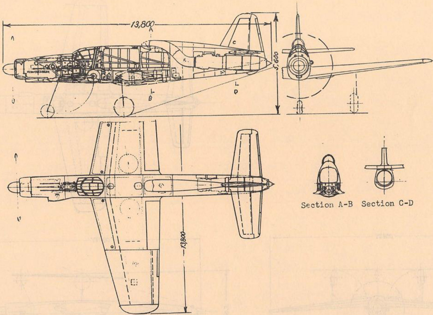
Fig. 2 - Longitudinal Section
